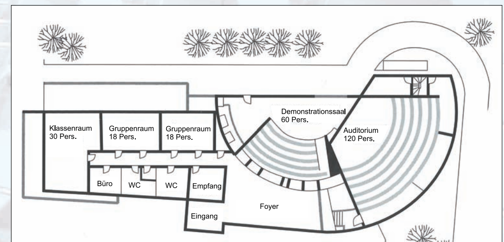
Seminarzentrum TFB AG im Grundriss
